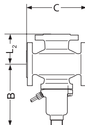
VFG 33/34 DN 25 - 125
