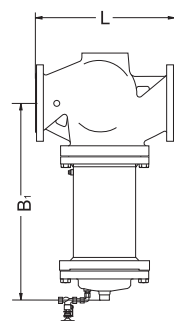
VFG, VFGS 2 DN 150 - 250 с удлинителем штока для t > 150\text{ }^{\circ}\text{C}
