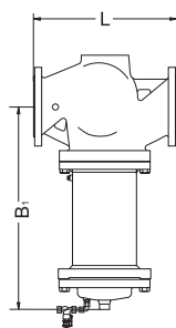
VFG DN 150 - 250 с удлиненным штоком для t > 150^{\circ}\text{C}
