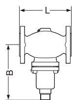
VFG DN 15 - 125
