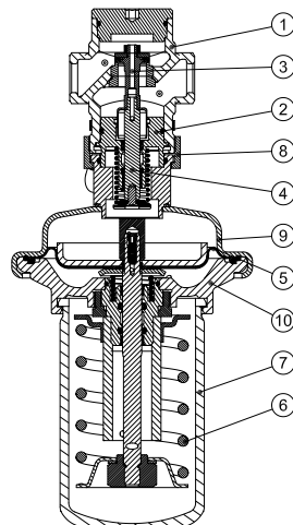
AVPA
