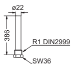
Погружная гильза (Примечание: R1 коническая наружная резьба по DIN 2999)
