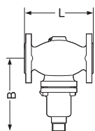
VFG DN 15 - 125
