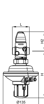
AVPQ DN 15 - 50 \Delta p = 0,2 - 1,0 бара
