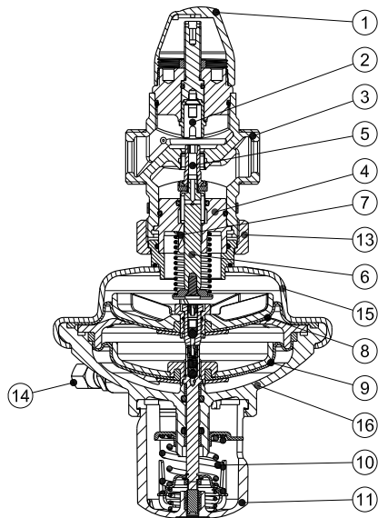
AVPQ (0,2 - 1,0 бар) – установка на обратном трубопроводе
