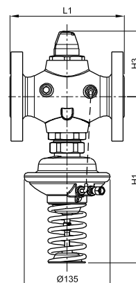
AVPQ DN 32 - 50 \Delta p = 0,3 - 2,0 бара
