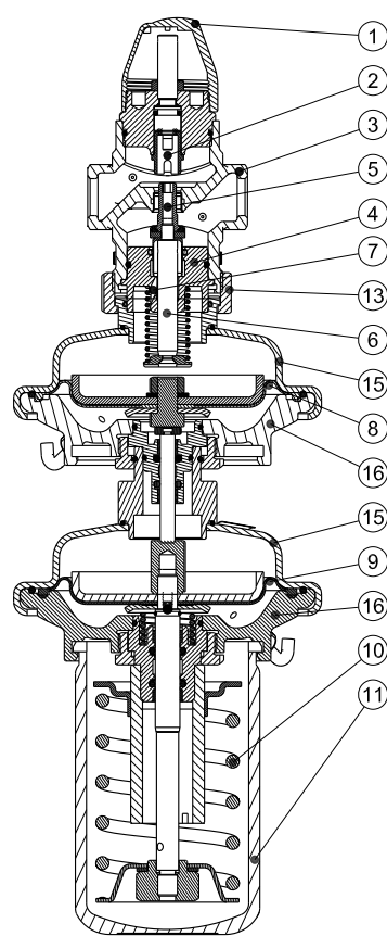
AVPQ 4 – установка на подающем трубопроводе
