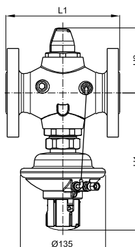
AVPQ DN 32 - 50 \Delta p = 0,2 - 1,0 бара
