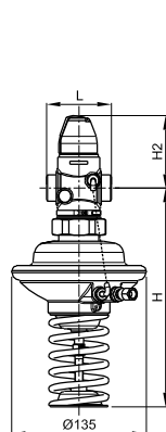
AVPQ DN 15 - 50 \Delta p = 0,3 - 2,0 бара
